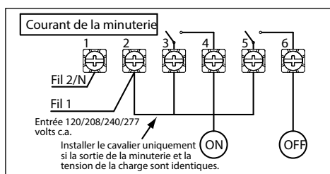
La minuterie ET8215 est configurée pour une impulsion unipolaire unidirectionnelle (SPST) avec le cavalier réglé sur PUL
