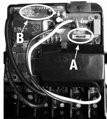
Vue arrière
