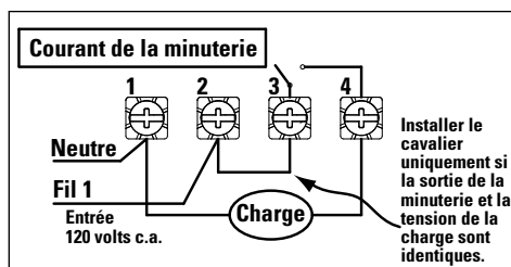
ET8015 configuré pour unipolaire unidirectionnel (SPST), charge 120 V c.a.
