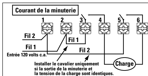
La minuterie ET8215 est configurée pour une communication de charge 240 V c.a. bipolaire unidirectionnelle (DPST) avec le cavalier réglé sur SIM
