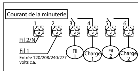
La minuterie ET8215 est configurée pour une communication bipolaire unidirectionnelle (DPST) avec le cavalier réglé sur SIM
