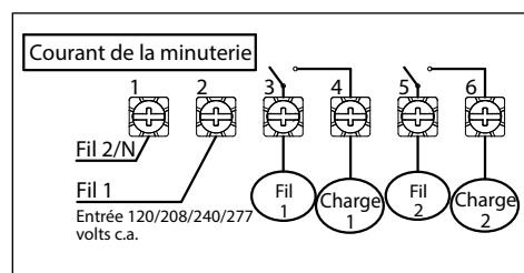
La minuterie ET8215 est configurée pour deux impulsions unipolaires unidirectionnelles (SPST) avec le cavalier réglé sur IND
